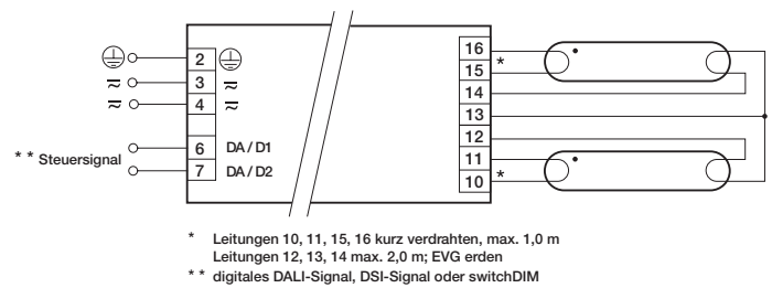
PCA T8 EXCEL one4all Ip x1tec II 2x14–80 W
